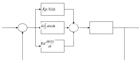
Gambar 3. Kontroler PID
