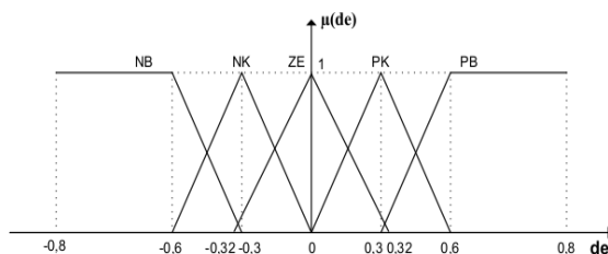
Gambar 3. Fungsi Keanggotaan dan Variabel Linguistik untuk e
