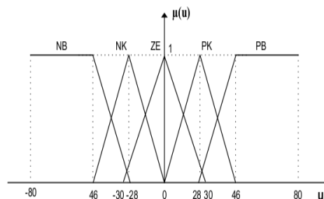
Gambar 4. Fungsi Keanggotaan dan Variabel Linguistik untuk de
