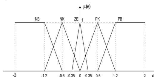
Gambar 5. Fungsi Keanggotaan dan Variabel Linguistik untuk u
